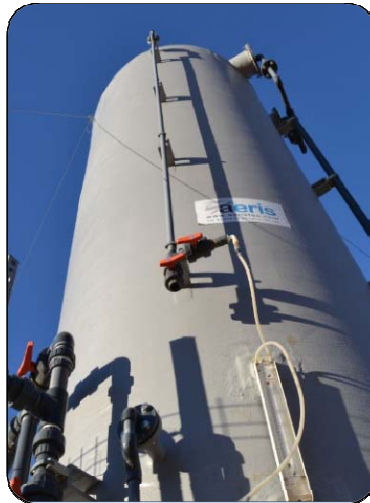
Biorreactor AERIS-SOX para la desulfuración de biogás
